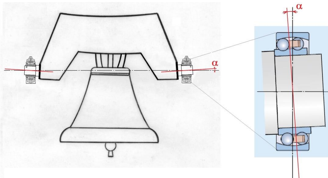
Alignement automatique du roulement sur la bague sphérique
